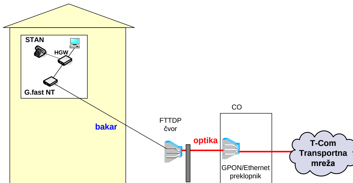
Slika 36a. Način realizacije FTTPD koncepta sa G.fast tehnologijom u pristupnoj mreži
