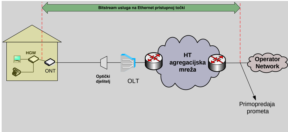
Slika 5. Veleprodajni širokopojasni pristup za pružanje Internet usluge na Ethernet razini kod pristupa preko FTTH rješenja
