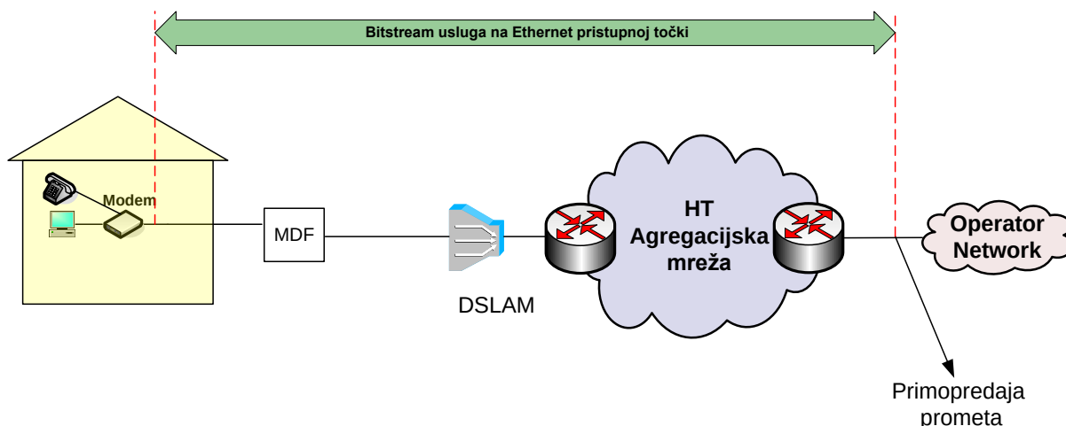
Slika 15. Veleprodajni širokopojasni pristup za pružanje VoIP usluge na Ethernet razini u slučaju kada krajnji korisnik ostvaruje Osnovni pristup mreži putem usluge Operatora korisnika
