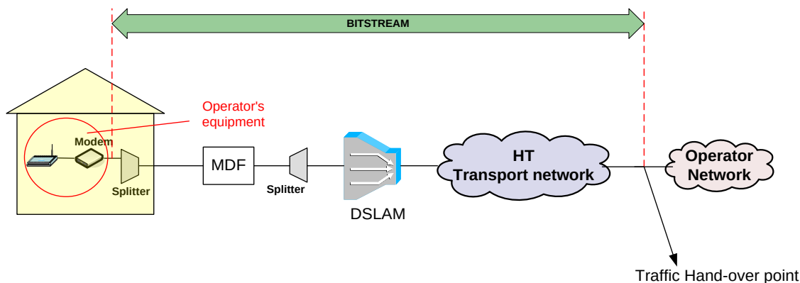
Slika 32. Koncept posebnog virtualnog kanala za Podatkovnu uslugu
