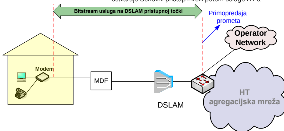
Slika 7. Veleprodajni širokopojasni pristup za pružanje Internet usluge na DSLAM razini u slučaju kada krajnji korisnik ostvaruje Osnovni pristup mreži putem usluge HT-a
