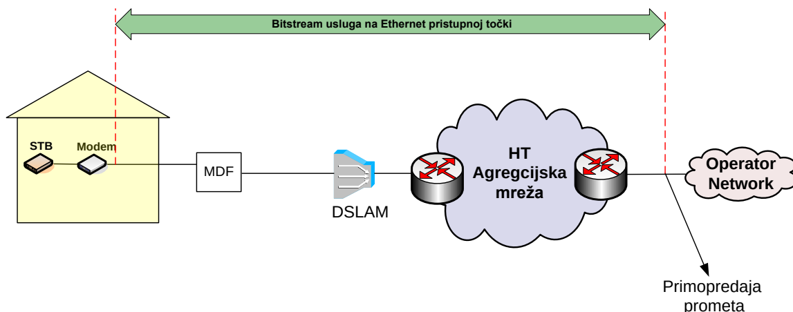
Slika 25. IPTV usluga na Ethernet razini putem ADSL/VDSL tehnologije u slučaju kada krajnji korisnik ostvaruje Osnovni pristup mreži putem usluge Operatora korisnika
